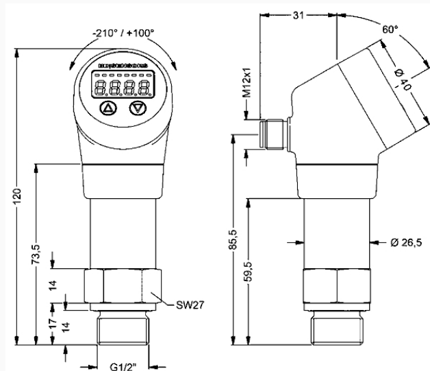
Elektronischer Druckschalter EDS 10
