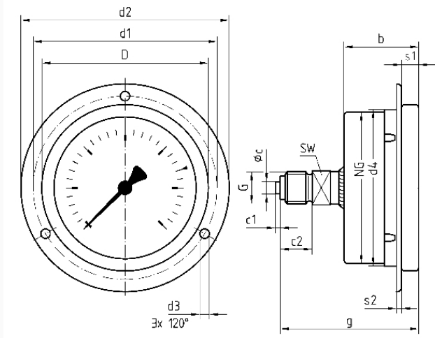
NG 63 – Anschluss axial exzentrisch, 3-Lochfrontflansch
