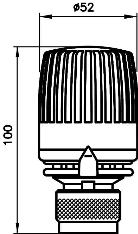
Thermostat-Regelkopf 323 KD mit festem Fühler, Danfoss-Klemmanschluss
