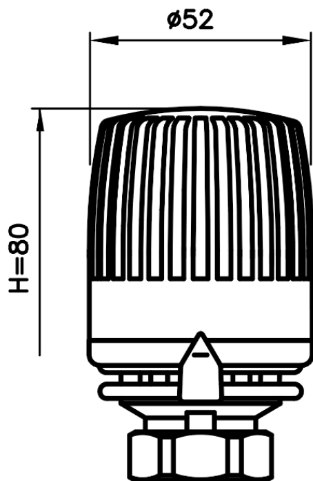
Thermostat-Regelkopf 323 mit festem Fühler
