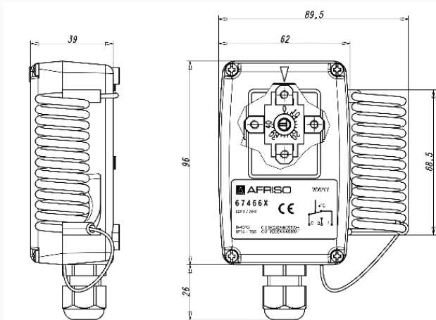
GRT/7HT, radial, Verstellung innenliegend (0-40 °C)
