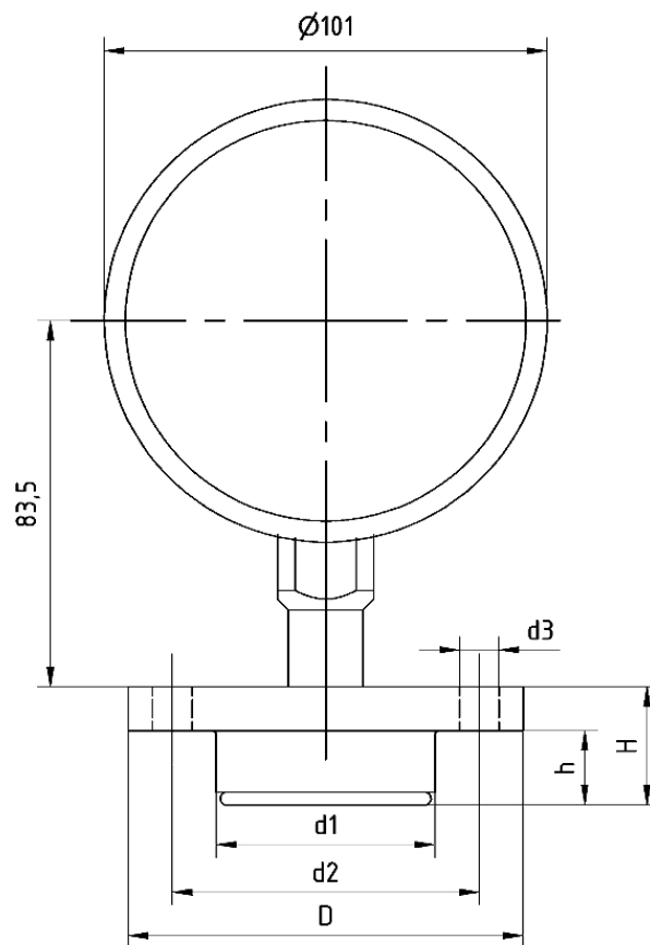
Manometer NG 100 mit MD 56
