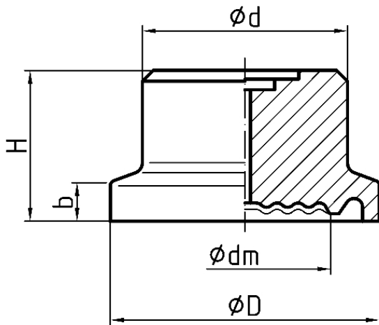
Typ MD 60 - Clamp-Anschluss 3/4" ISO 2852
