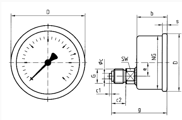
NG 50 – Anschluss axial exzentrisch
