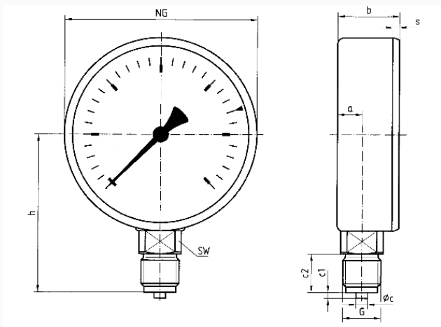
Masse (mm)
