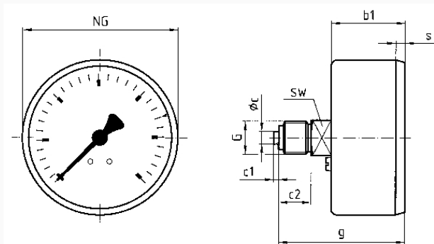
NG 40/50/63 – Anschluss axial
