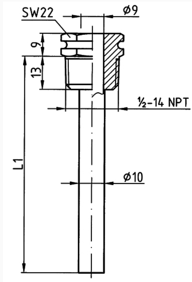
Tauchhülse 1/2" 9 x 10 mm
