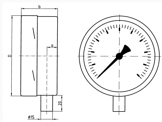
Anschluss radial
