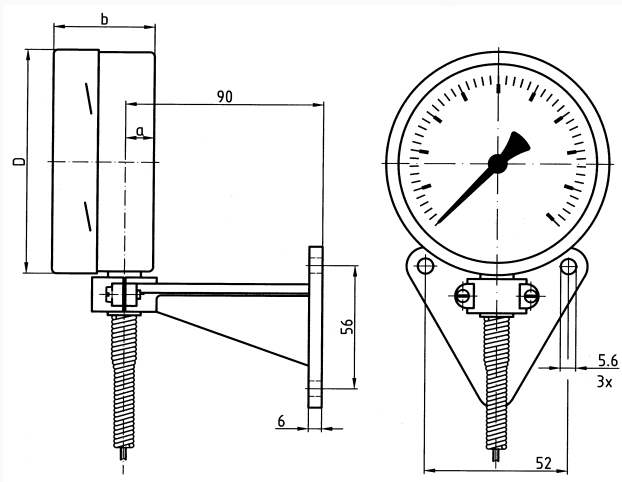
Ausführung mit Fernleitung und Wandhalterung
