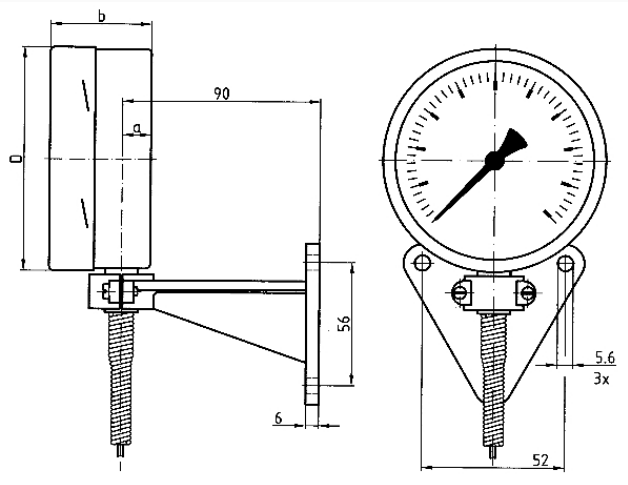
Masse (mm)
