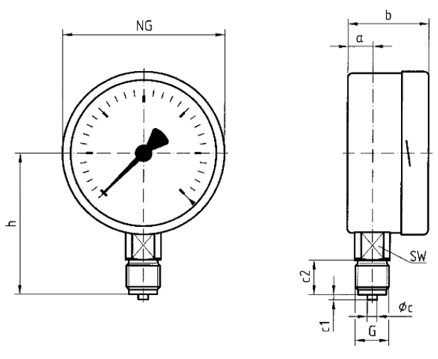
Masse (mm)
