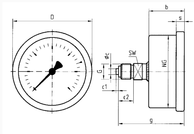
Masse (mm)
