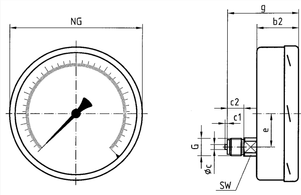
Maße (mm)
