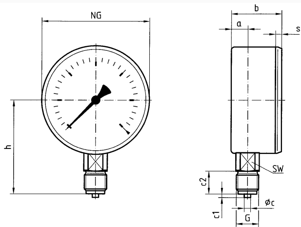
Anschluss radial
