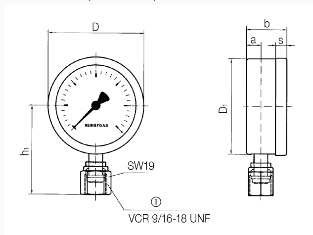
Anschluss radial, 9/16-18 UNF, mit Überwurfmutter
