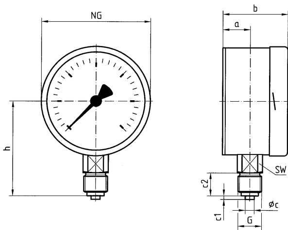
Maße (mm)
