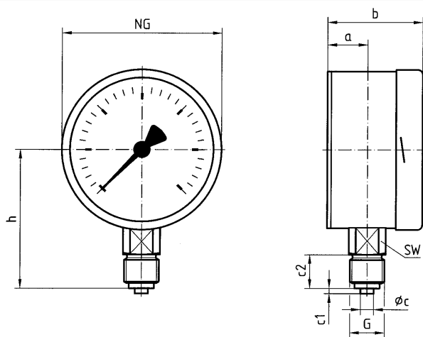
Maße (mm)
