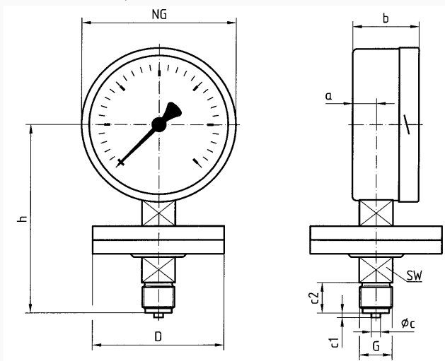
Maße (mm)
