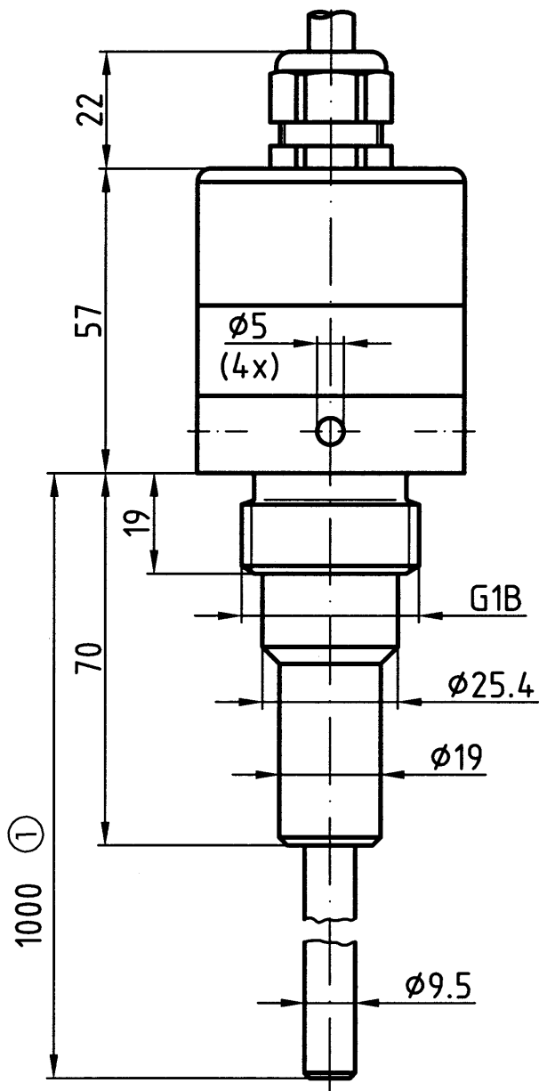
Einstabsonde LST 23
