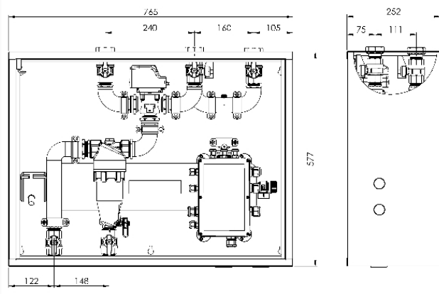
Masse (mm)
