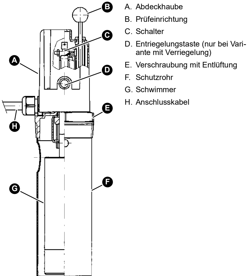
Abbildung 2: WMS-WP6 R2 mit kurzem Schutzrohr
