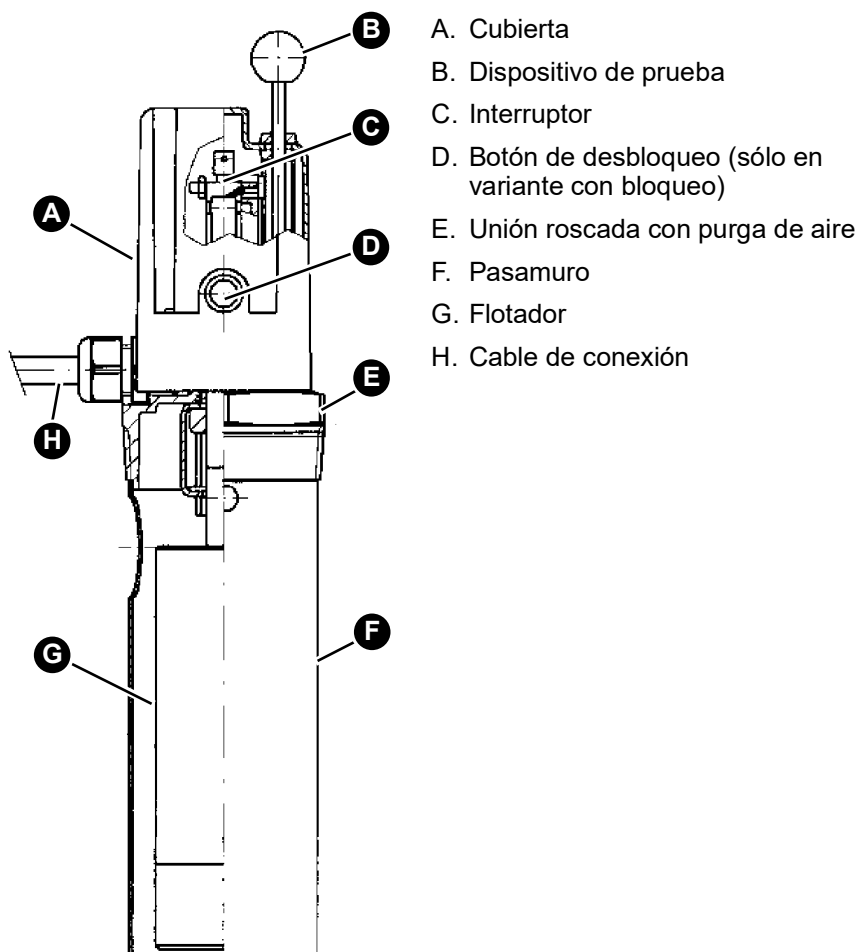
Figura 2: WMS-WP6 R2 con pasamuro corto
