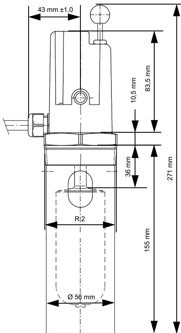
Figura 4: WMS-WP6 R2 con pasamuro corto
